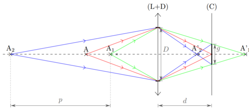
FIGURE 1 : Schéma illustrant la notion de mise au point et profondeur de champ. Le diaphragme et la lentille sont confondus. La mise au point d est réalisée pour l'objet A situé à la distance L de l'objectif. Tous les objets situés entre A_1 et A_2 auront une image sur le capteur de taille inférieure ou égale au grain g , ces images seront toutes nettes. La profondeur de champ p est la distance entre ces deux points.
